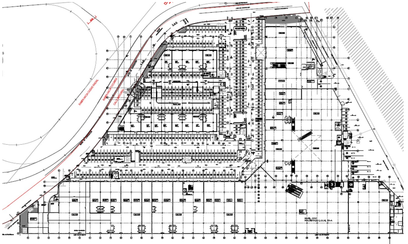
PLANTA ARQUITECTONICA NIVEL 000 11/1/2001
