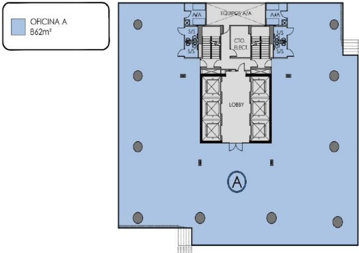
PLANTA TIPICA DE OFICINAS - NIVEL 3000@ 3500
