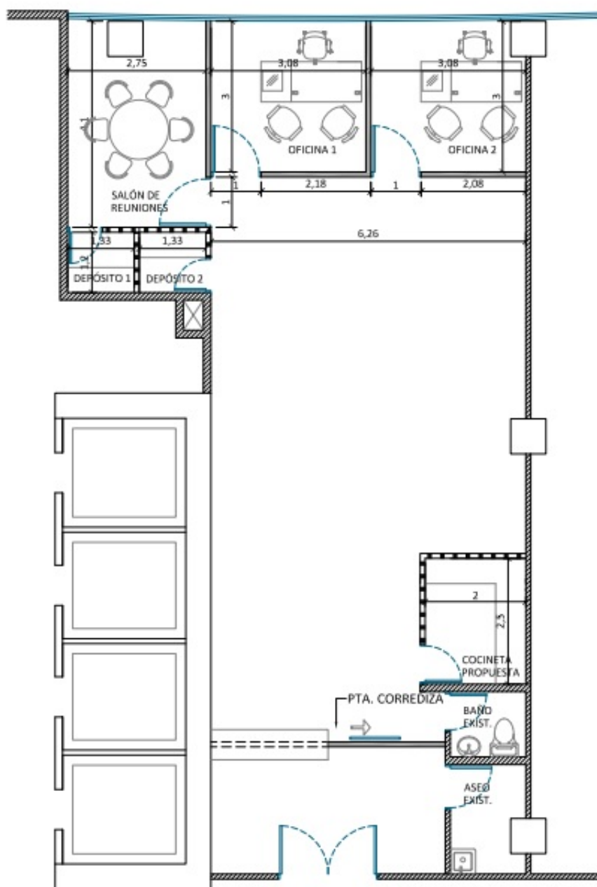
PLANTA ARQUITECTÓNICA PROPUESTA
