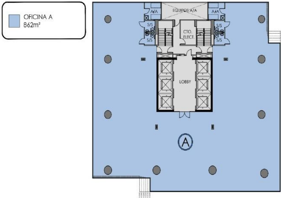
PLANTA TÍPICA DE OFICINAS - NIVEL 3000@ 3500
