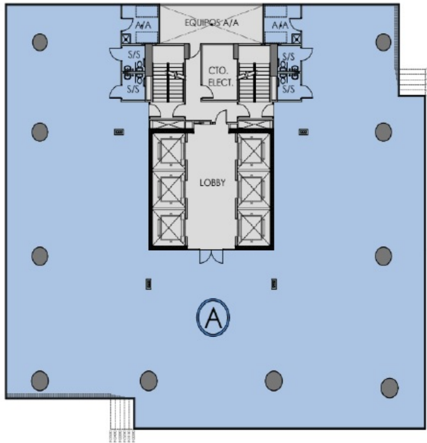
PLANTA TIPICA DE OFICINAS - NIVEL 3000@ 3500
